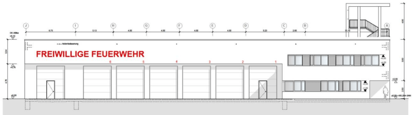
Ansicht Norden
